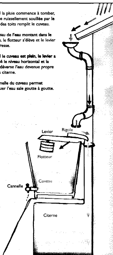
13 - Exemple d'un système séparateur de récupération de l'eau de pluie
